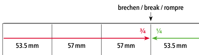
Quersteg | Transversal divider Élément de séparation transversal
